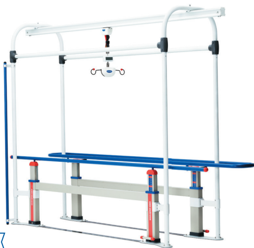
昇降式平行棒 標準型 オーバーヘッドセット GH-2650-S2 ※上記は起立トレーニング用縦手すりと免荷量表示計のオプションつきです。
